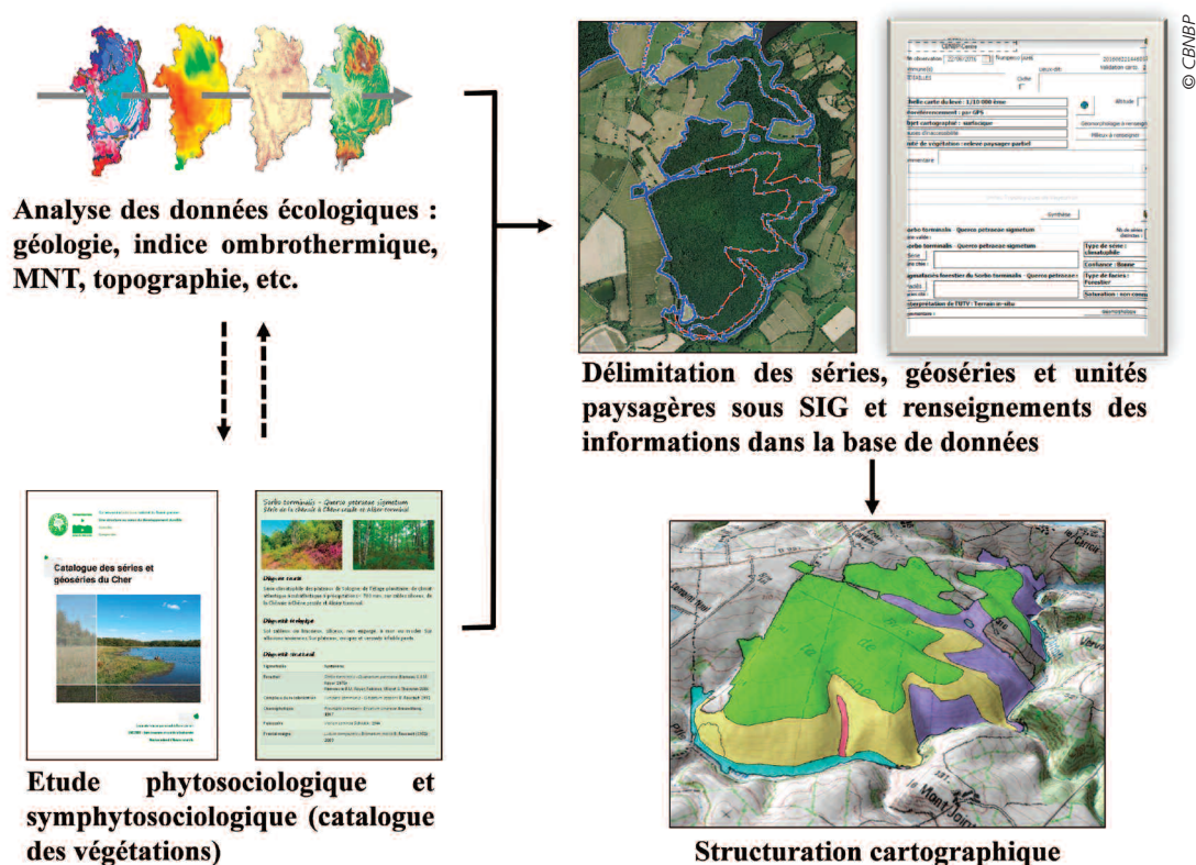
Figure 9. Les différentes phases de l'opération de cartographie in situ .
