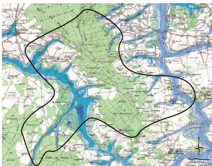
Figure 16. Fond environnemental, couche des milieux humides et linéaires de cours d'eau.
