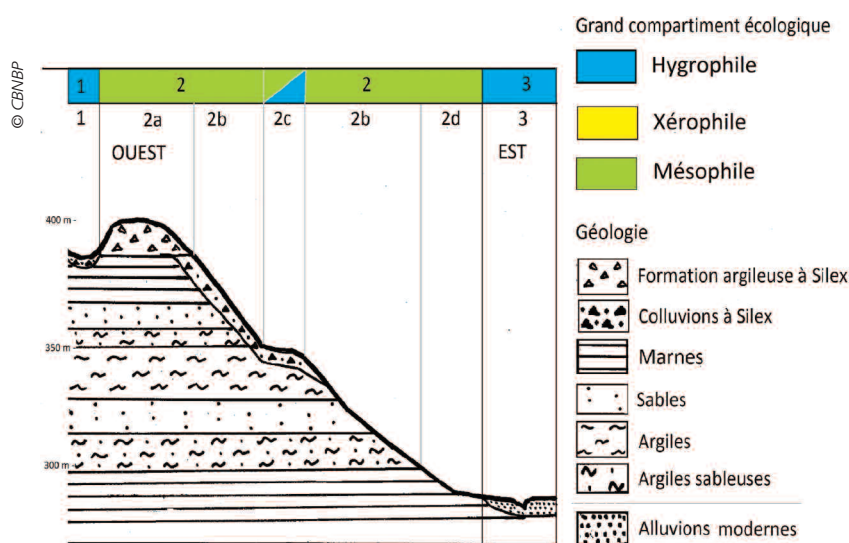
Figure 15. Transect d'organisation de la végétation en fonction de la géologie et de la topographie sur les communes de la Chapelotte et de Sens-Beaujeu (au sud du Pays-Fort). Ce transect ne détaille pas toutes les UTV du Pays-Fort.
