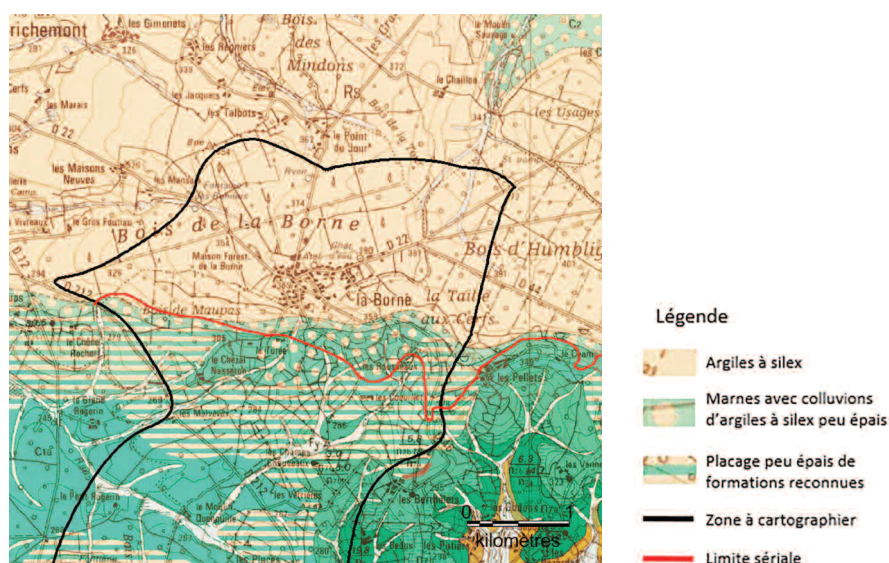
Figure 21. Cartographie de la limite entre le Vaccinio myrtilli – Quercu petraeae sigmetum prov. et le Melico uniflorae – Fago sylvaticae sigmetum prov. Source : fond géologique du BRGM au 1:50 000.
