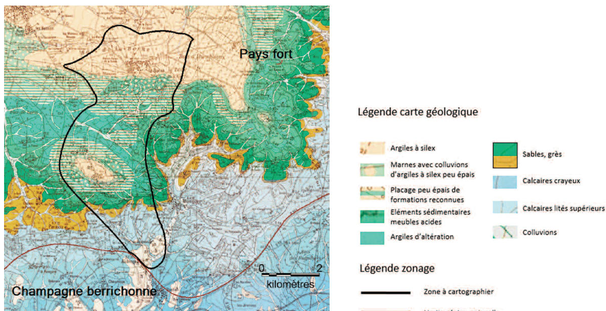
Figure 19. Zone à cartographier sur les communes de la Borne et de Henrichemont (sud du Pays-Fort), fond géologique du BRGM au 1:50 000.
