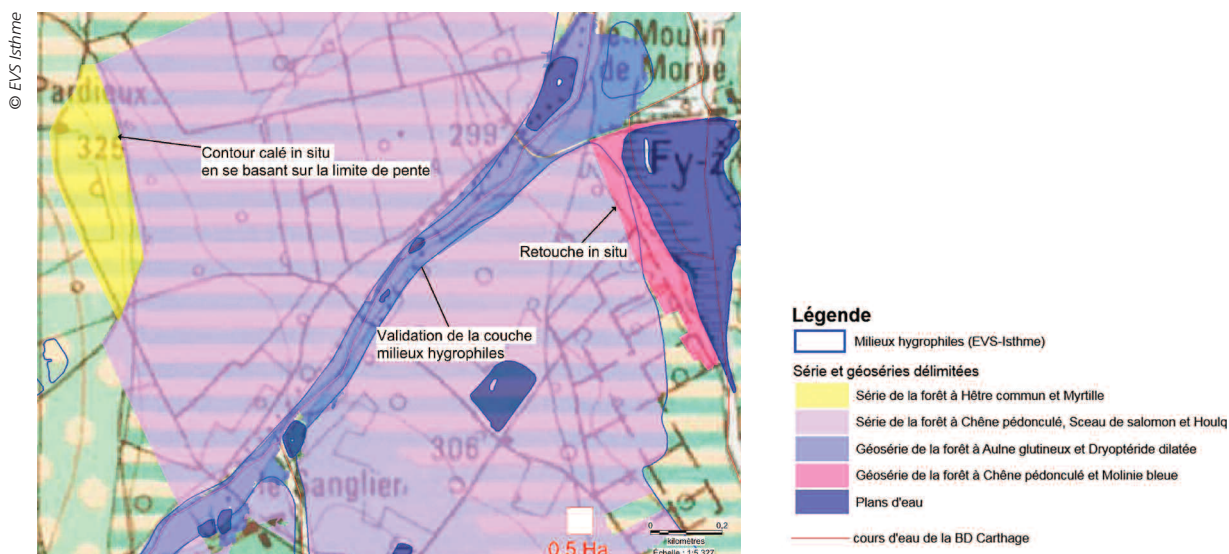
Figure 18. Exemple de délimitation de séries et petites géoséries dans les compartiments humides.
