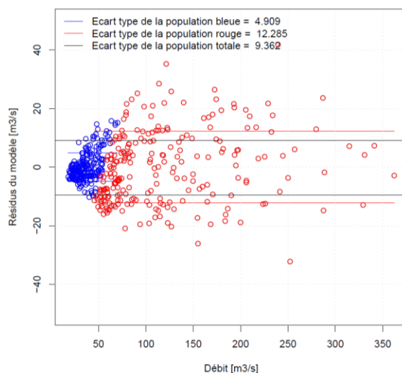
Figure 3 : Evolution des deux sous populations des résidus en fonction du débit – Valeurs des écarts types respectifs.
