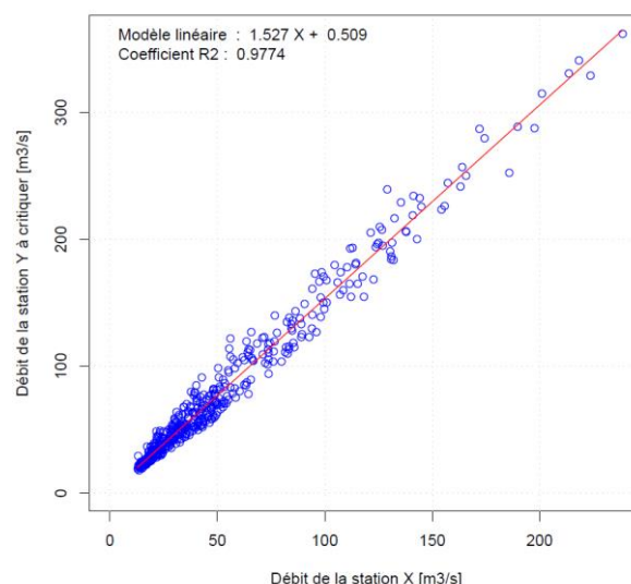
Figure 1 : Modèle linéaire entre la variable à expliquer (Données mensuelles de la station Y) et la variable d'explication (Données mensuelles de la station X)
