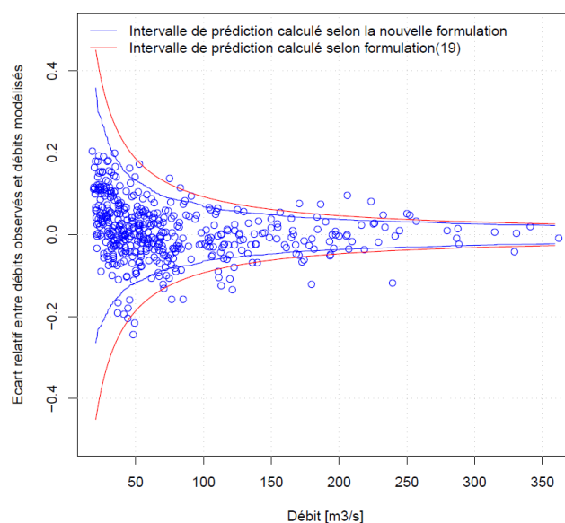
Figure 10 : Ecarts relatifs entre les débits modélisés et les débits observés munis des intervalles de prédiction au seuil de confiance de 95% calculés de deux façons différentes pour le modèle linéaire double
