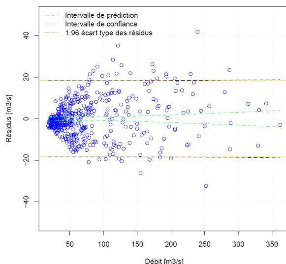
Figure 2 : Représentation des résidus du modèle linéaire en fonction du débit – Intervalle de confiance et Intervalle de prédiction
