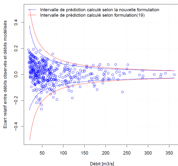
Figure 11 : Ecart relatif entre les débits modélisés et les débits observés munis des intervalles de prédiction au seuil de confiance de 95% calculés de deux façons différentes pour le modèle linéaire simple avec comme variable explicative (X + Z)
