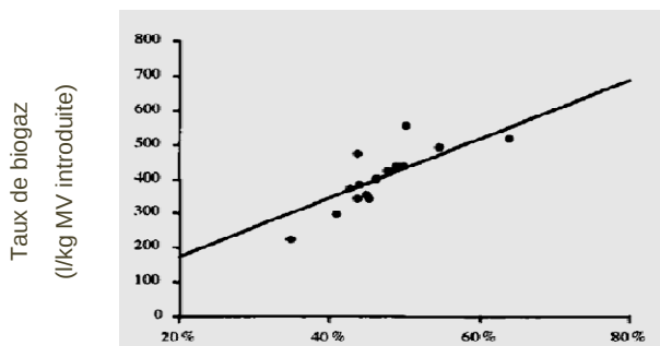
Figure 4 : Relation entre le taux de biogaz (par kg de MV introduite) et le pourcentage de MV détruites (Barber, 2005)
