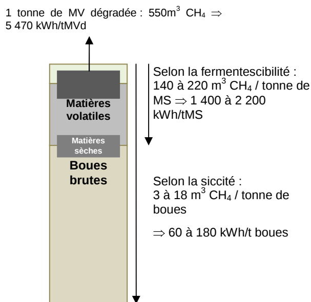
Figure 5 : Estimation des productions énergétiques lors de la digestion des boues
