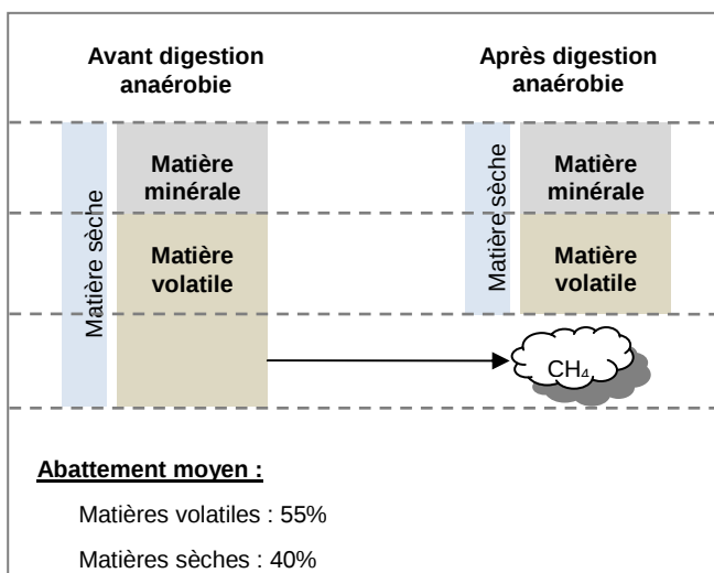
Figure 3 : Dégradation de la matière sèche lors de la digestion anaérobie des boues
