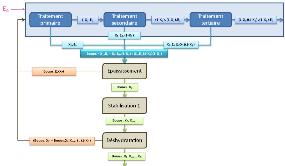
Figure 1 : Représentation schématique de l'équation générale des retours en tête
