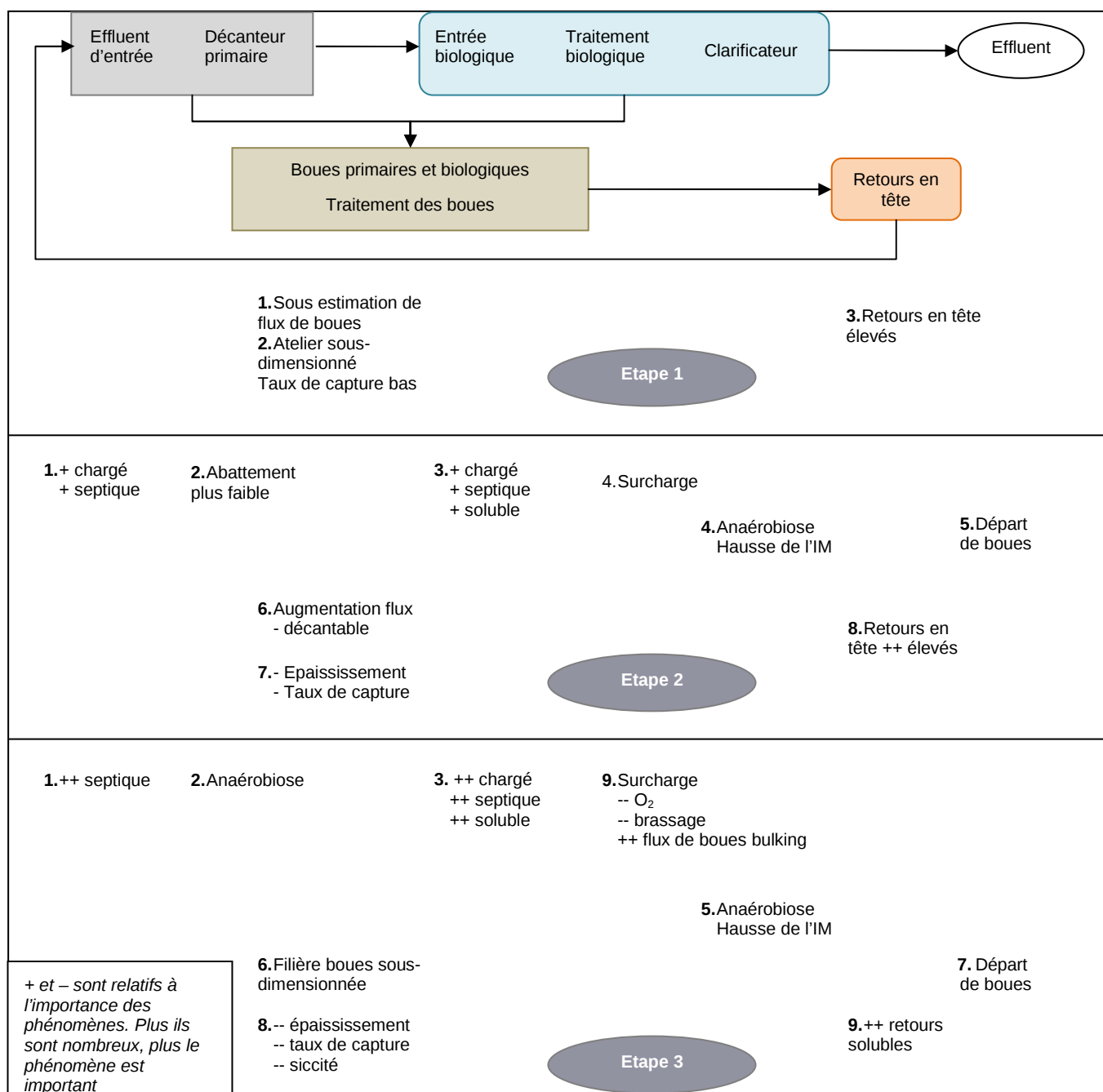
Figure 2 : Scénarios de dysfonctionnements dus aux retours en tête (Grulois et al., 1993)
