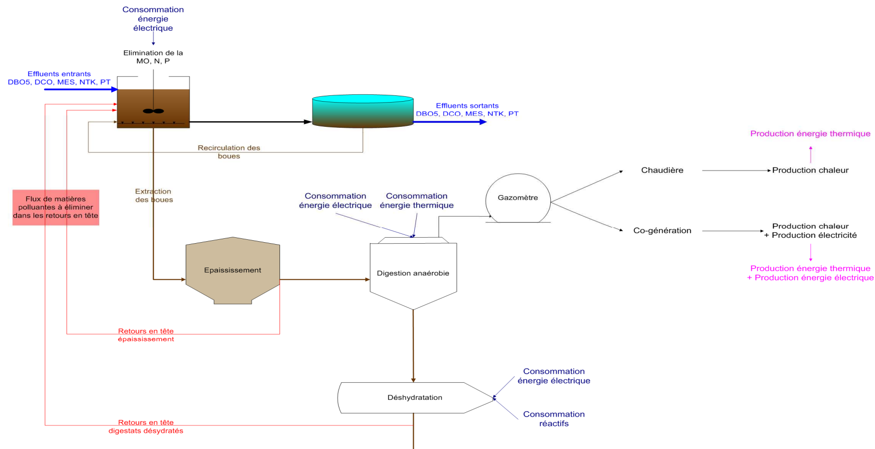
Figure 9 : Représentation schématique des postes à étudier sur les 5 STEU afin d'évaluer les impacts de la digestion anaérobie sur les performances de la STEU
